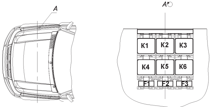
Рис. 2. Реле и предохранители:
